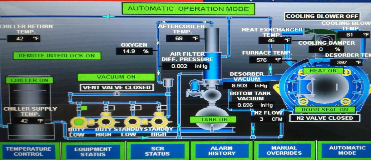
THERMAL DESORBER (MR-15EX)
